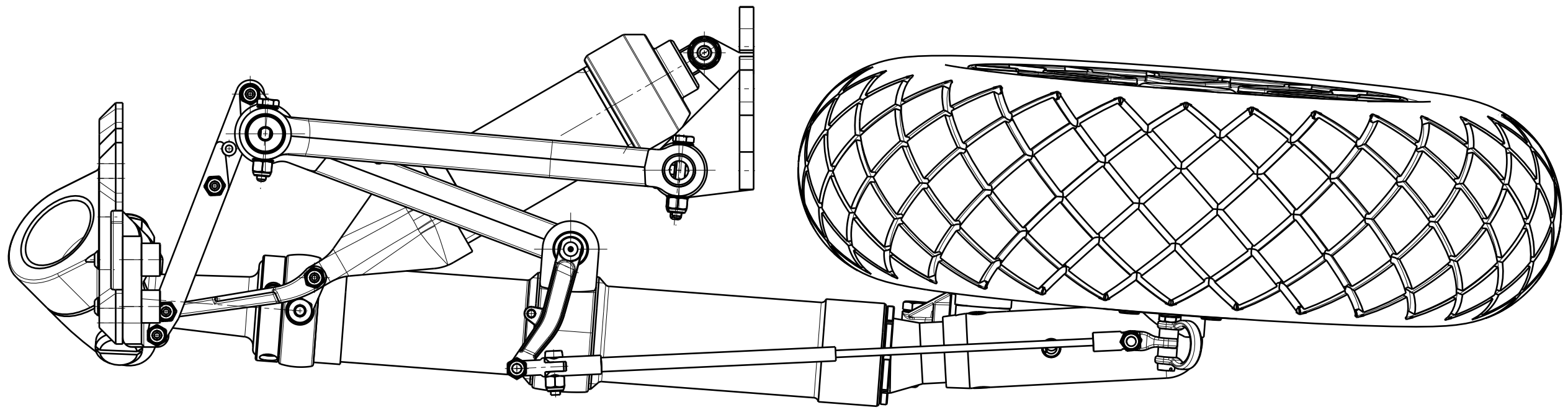
Vue de face Echelle : 1:1
