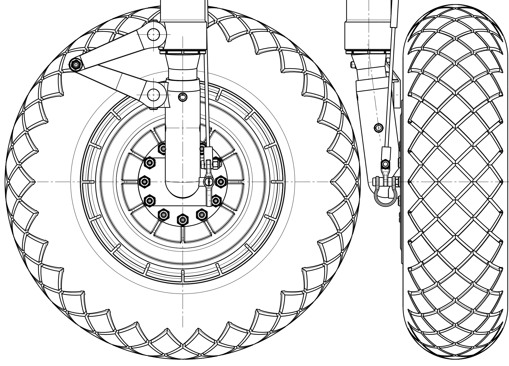
Vue de face Echelle : 1:1
