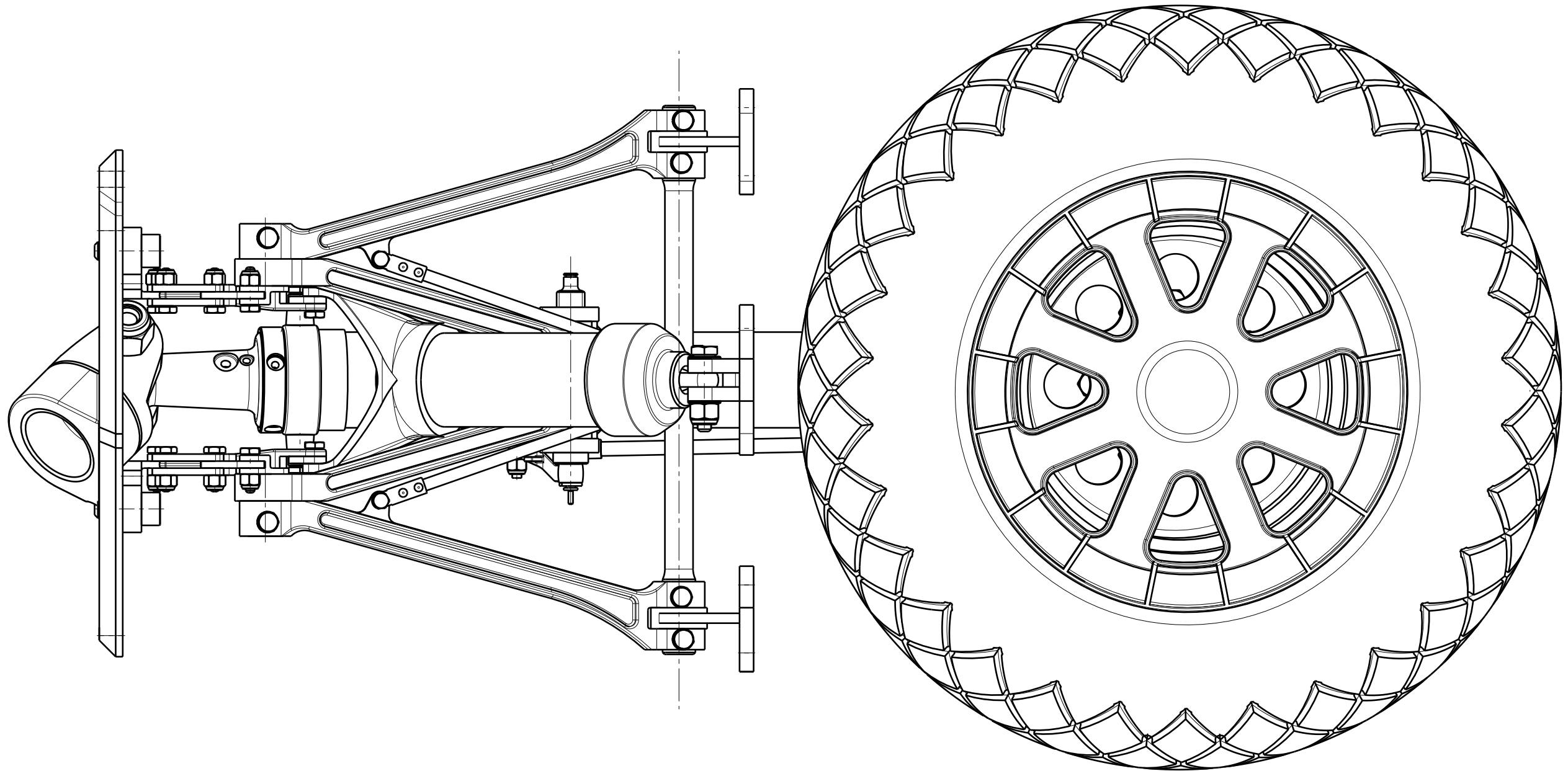
Vue de face Echelle : 1:1
